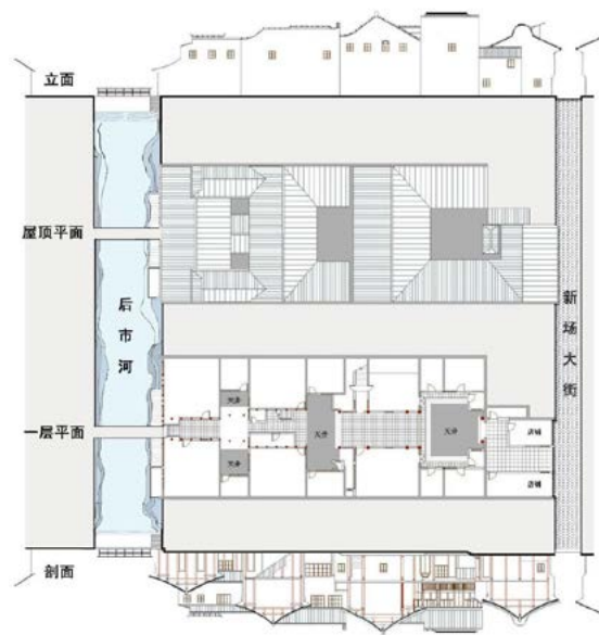
张氏宅第平、立、剖面示意图 典型的前街后河传统宅园
